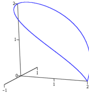
Curva de Viviani
