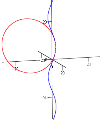
Circunferencia Oscultriz
