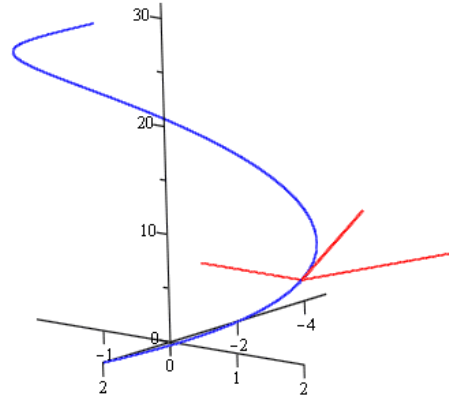
Triedro de Frenet
