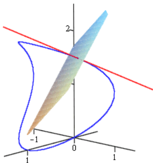
Recta tangente y plano normal
