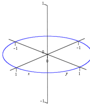
Circunferencia
